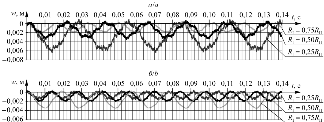
Рис. 3. Изменение величины прогиба в центральной точке пакета сталь – фторопласт-4 – сталь с уширением ( a ) и сужением ( b ) в центральной части
