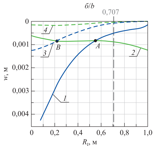
Рис. 8. Изменение прогиба в центральной точке пакета сталь – фторопласт-4 – сталь при динамическом (а) и квазистатическом (б) деформировании: 1, 2 – нагружение участка I в пластине с уширением и сужением в центральной части соответственно; 3, 4 – нагружение участка II в пластине с уширением и сужением в центральной части соответственно
