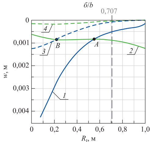
Рис. 9. Изменение прогиба в центральной точке пакета сталь – ПС-1 – сталь при динамическом (а) и квазистатическом (б) деформировании: 1, 2 – нагружение участка I в пластине с уширением и сужением в центральной части соответственно; 3, 4 – нагружение участка II в пластине с уширением и сужением в центральной части соответственно
