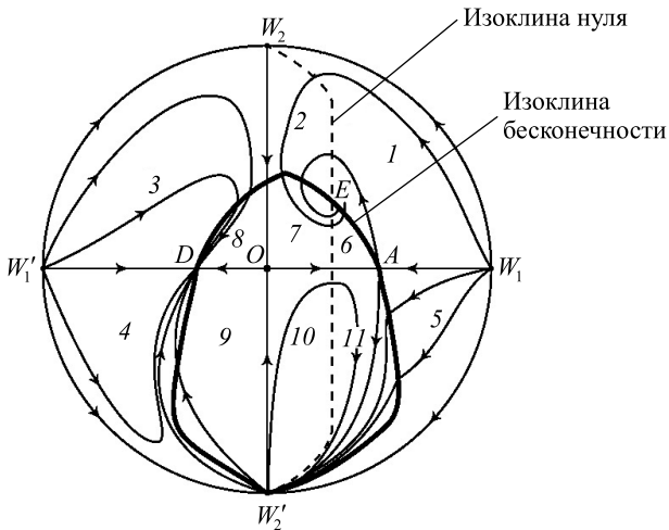
Рис. 1. Главные изоклины системы (1) в круге Пуанкаре
