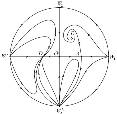
Рис. 2. Фазовый портрет системы (1) в условиях теоремы 1
