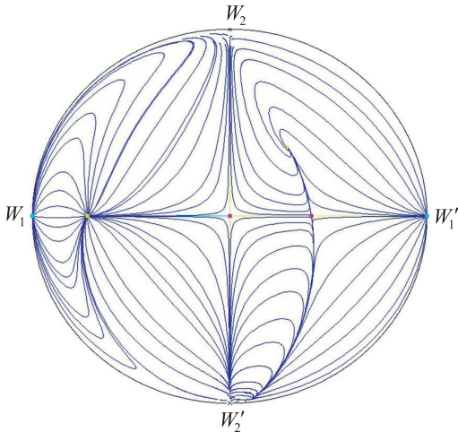
Рис. 3. Фазовый портрет системы (11)
