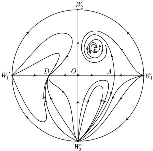
Рис. 6. Фазовый портрет системы (1) в условиях теоремы 4
