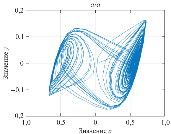
Рис. 1. Формы аттракторов для различных значений управляющего параметра \delta : a - \delta = 0,2 ; b - \delta = -0,4
