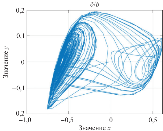
Рис. 1. Формы аттракторов для различных значений управляющего параметра \delta : a - \delta = 0,2 ; b - \delta = -0,4
