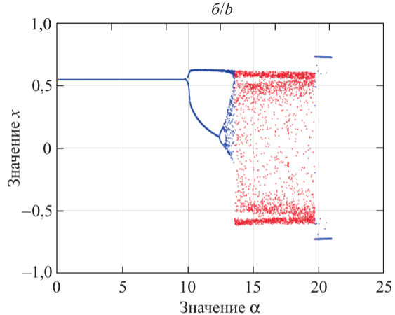
Рис. 3. Бифуркационные диаграммы для системы (1): a – при управлении по параметру \delta ; b – при управлении по параметру \alpha ( \delta = 0 )
