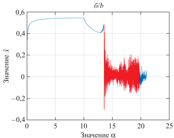
Рис. 4. Зависимость среднего арифметического значения первой переменной пространства состояний \tilde{x} от управляющего параметра: a – при управлении по параметру \delta ; b – при управлении по параметру \alpha ( \delta = 0 )
