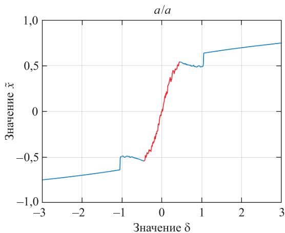
Рис. 4. Зависимость среднего арифметического значения первой переменной пространства состояний \tilde{x} от управляющего параметра: a – при управлении по параметру \delta ; b – при управлении по параметру \alpha ( \delta = 0 )
