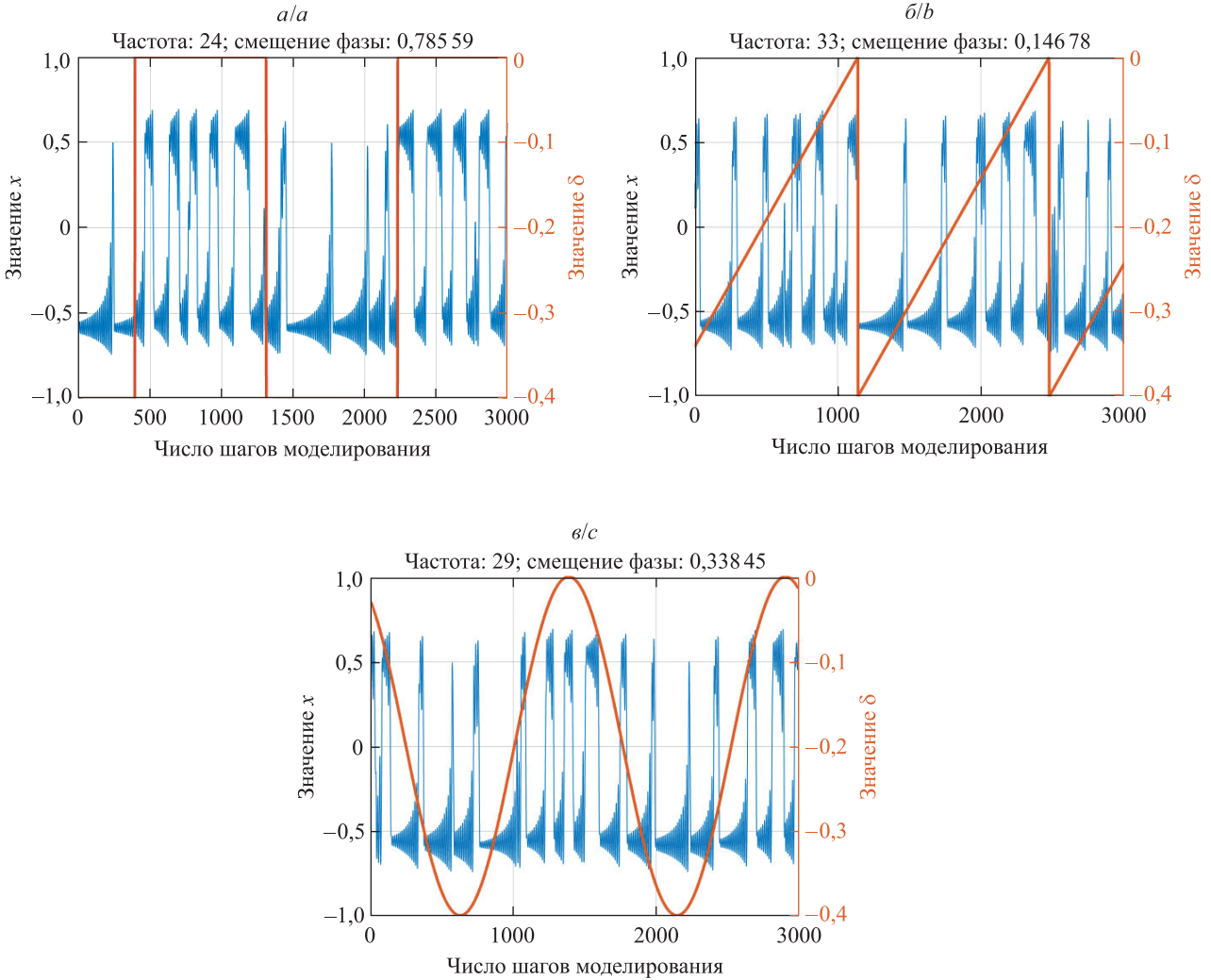
Рис. 7. Влияние тестовых сигналов (линии красного цвета) на динамику осциллятора: а – квадратный сигнал; б – треугольный сигнал; в – синусоидальный сигнал Fig. 7. The dynamic of the oscillator under the influence of the different control signals (red lines): а – square signal; б – triangle signal; в – sinusoidal signal
