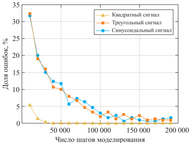
Рис. 9. Зависимость доли ошибок классификации от времени моделирования
