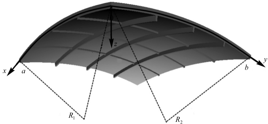
Рис. 1. Общий вид пологой оболочки двойкой кривизны, усиленной ребрами жесткости Fig. 1. General view of a shallow shell of double curvature, stiffened by ribs
