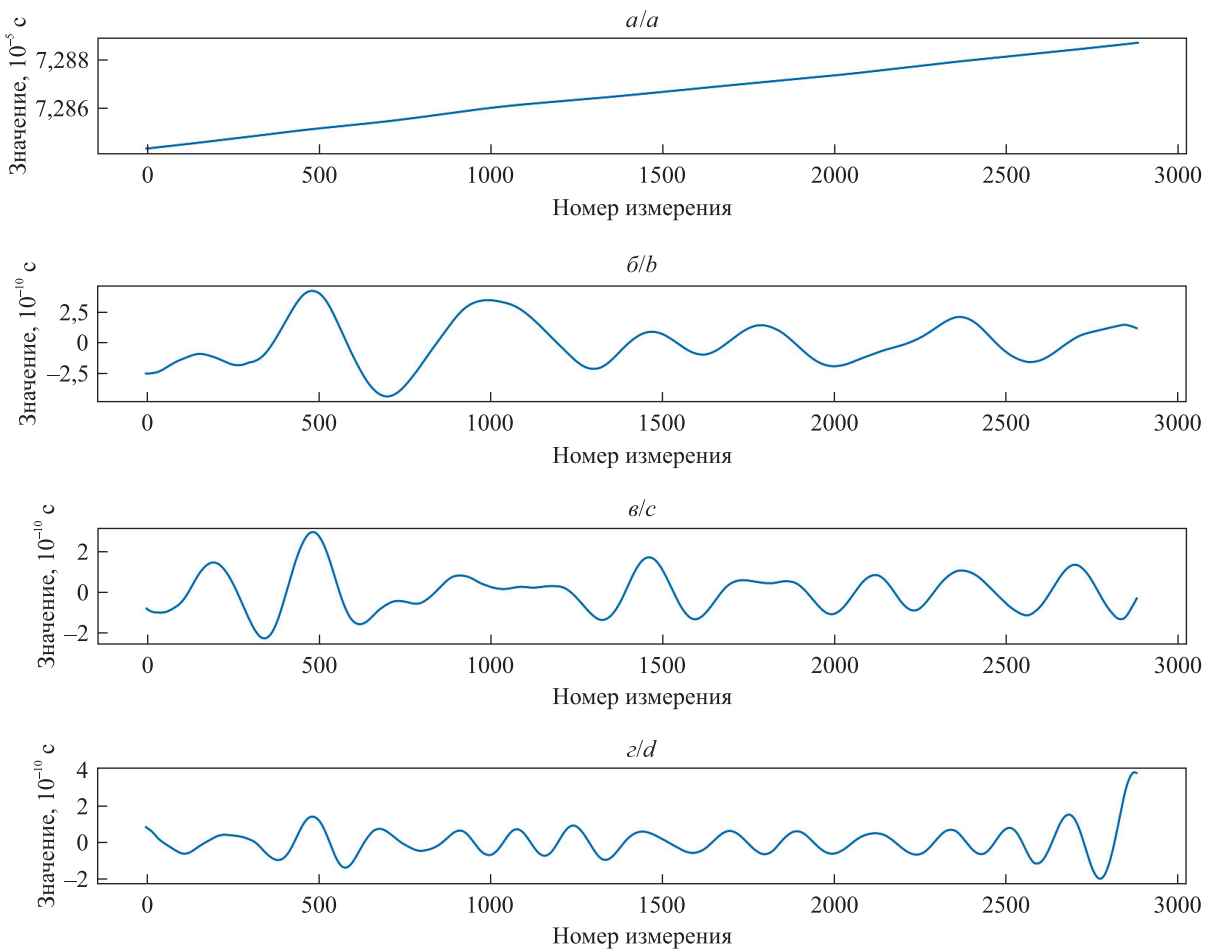
Рис. 2. Графическое изображение первых четырех компонент разложения исходного ряда значений РШВ: a – 99,996 %; b – 0,003 %; v – 0,000 2 %; z – 0,000 1 %
