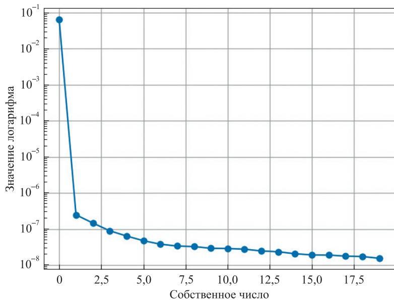
Рис. 3. Логарифмы собственных чисел сингулярного разложения траекторной матрицы
