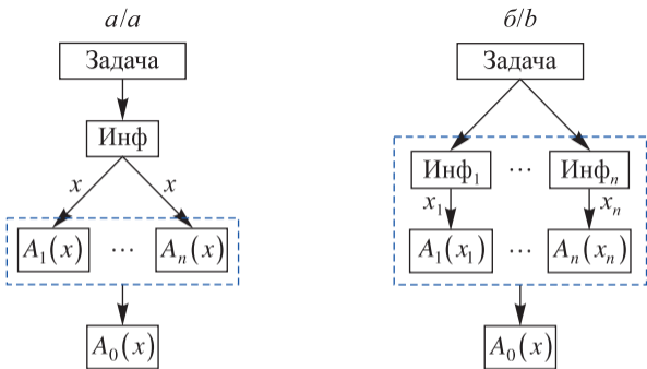
Рис. 1. Общая схема построения двухуровневых моделей распознавания (Инф – информация): a – вариант 1; б – вариант 2
