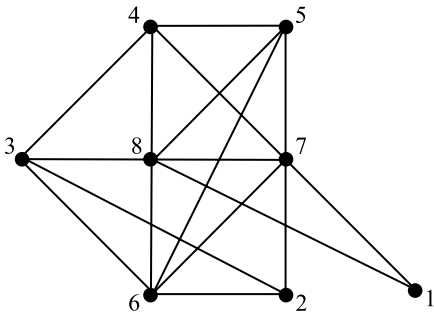
Рис. 1. Граф D_8
