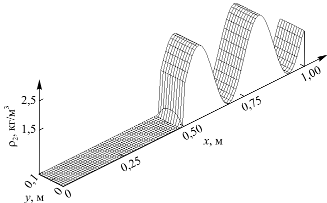
Рис. 2. Начальное пространственное распределение средней плотности дисперсной фазы
