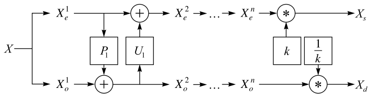
Рис. 2. Лифтинг-схема
