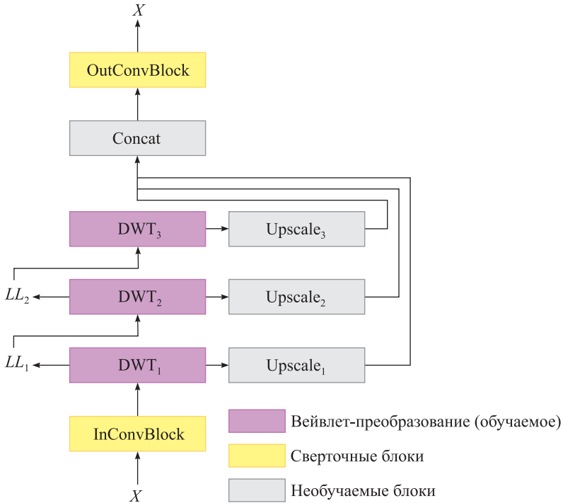
Рис. 3. Сверточный вейвлет-блок
