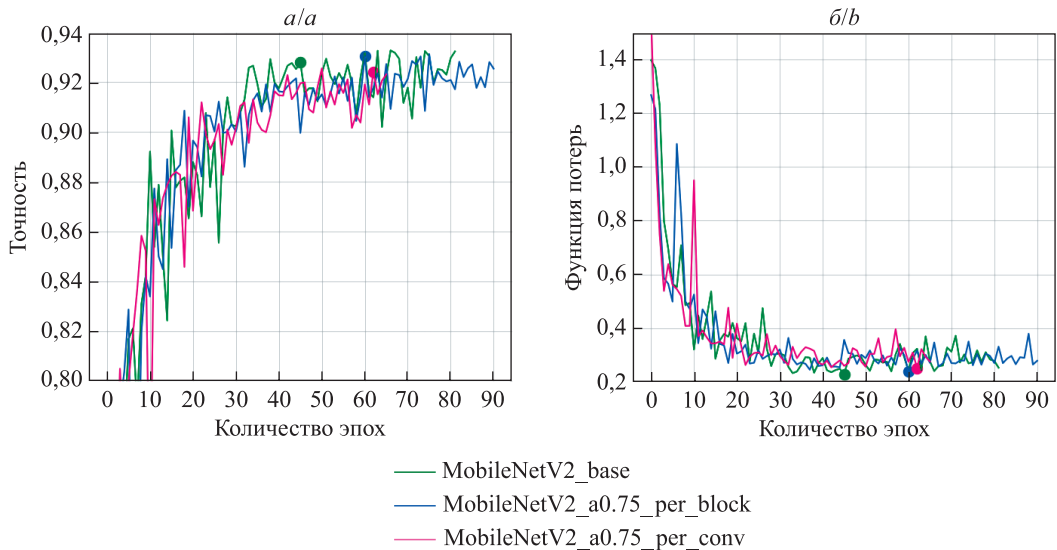
Рис. 9. Сходимость модели MobileNetV2 ( a – точность; b – функция потерь)
