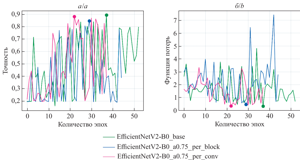
Рис. 10. Сходимость модели EfficientNetV2-B0 ( a – точность; b – функция потерь)
