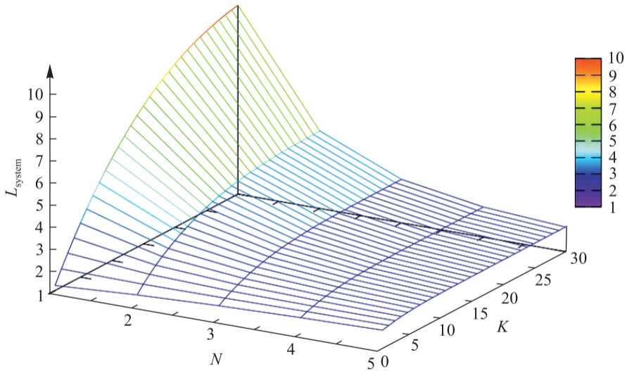
Рис. 2. Зависимость L_{\text{system}} от N и K
