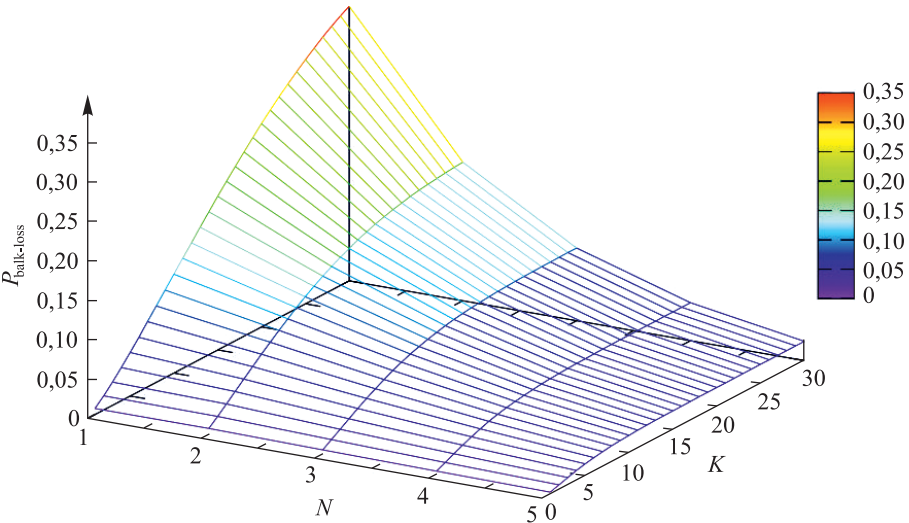
Рис. 8. Зависимость P_{\text{balk-loss}} от N и K Fig. 8. Dependence P_{\text{balk-loss}} on N and K
