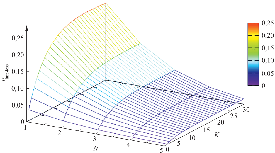
Рис. 9. Зависимость P_{\text{imp-loss}} от N и K
