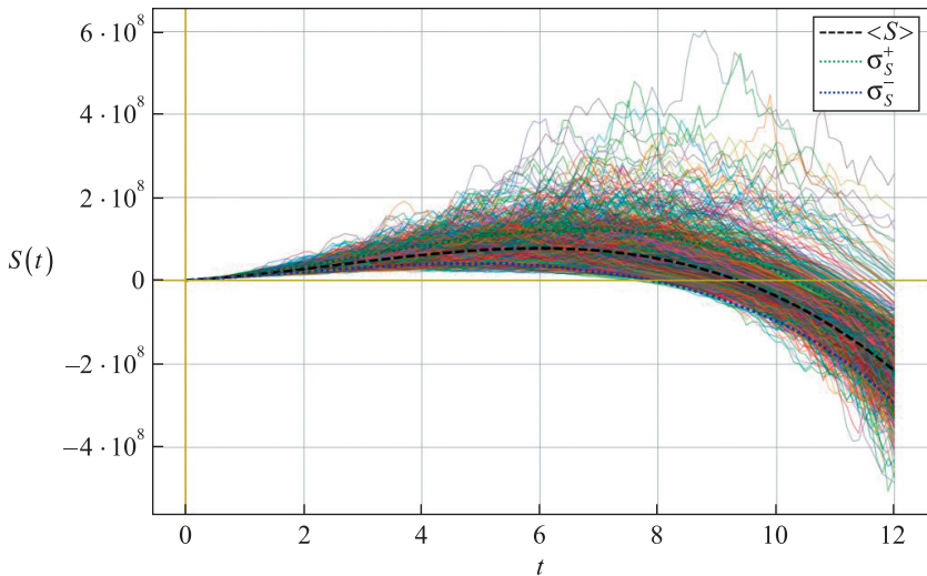
Рис. 8. Динамика прибыли финансовой пирамиды при линейном приросте клиентов, процентных расходах на рекламу и линейной волатильности (схема Рунге – Кутты 4-го порядка)
