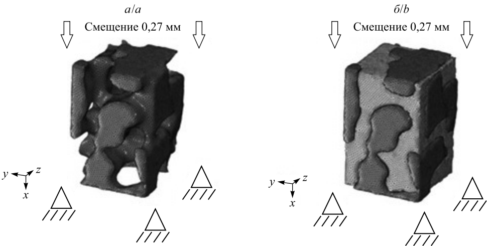
Рис. 1. Схема конечно-элементного моделирования механических испытаний на сжатие исследуемых образцов:
