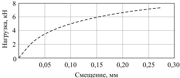
Рис. 2. Кривая зависимости смещения биокompозита от нагрузки при конечно-элементном моделировании испытаний на сжатие
