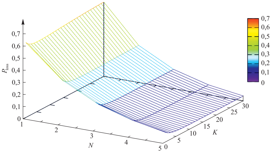
Рис. 11. Зависимость P_{\text{loss}} от N и K
