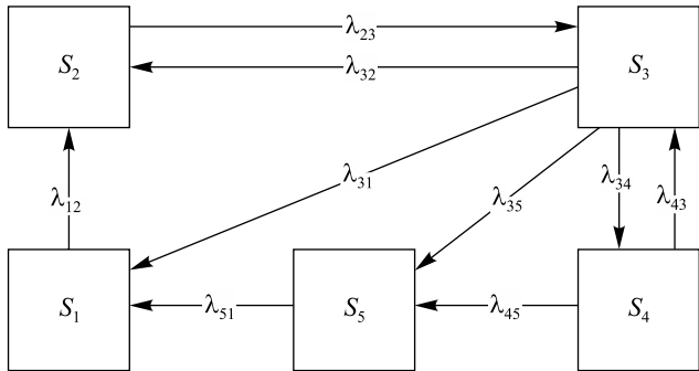
Рис. 1. Граф условных состояний системы передачи данных SDN
