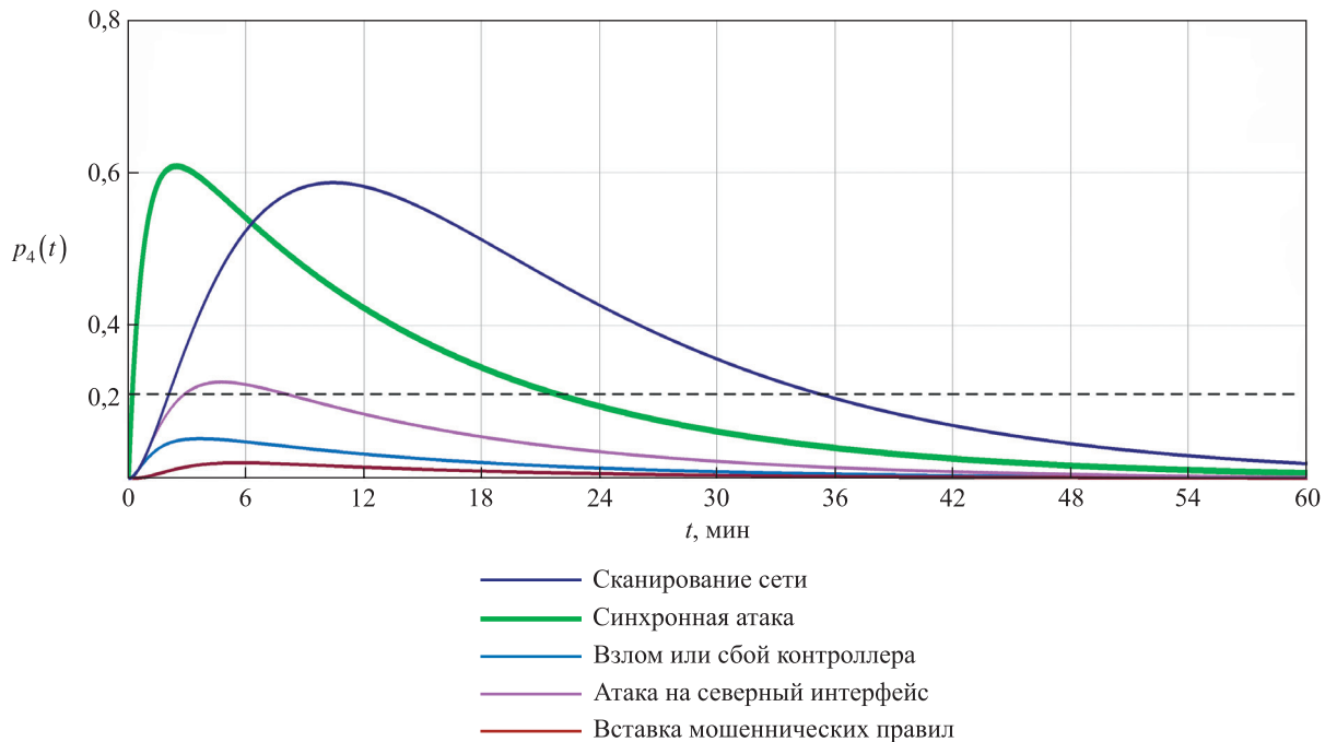
Рис. 5. Зависимость вероятности устойчивой работы SDN от времени реализации КА для структуры 3
