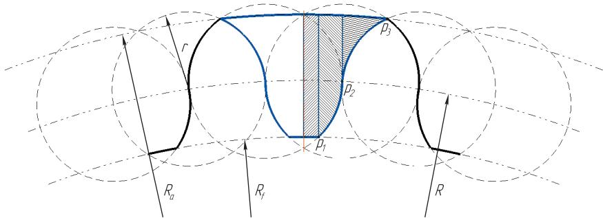
Рис. 2. Формирование формы зуба и вычисление площади впадины S_{\text{deep}}
