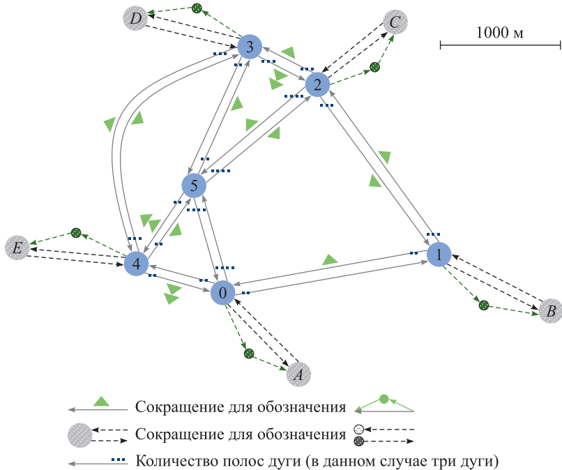
Рис. 3. Тестовый орграф дорожной сети
