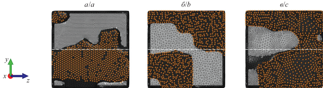
Рис. 5. Смещенные узлы сетки конечных элементов металлической составляющей трех образцов биокompозита кость – титан различной высоты (вид сверху): a – 4,5 мм; б – 4,0 мм; в – 3,5 мм
