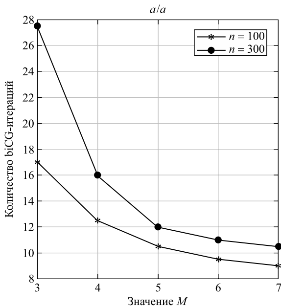
Рис. 2. Зависимость количества внешних итераций метода бисопряженных градиентов (biCG-итераций) (а) и удельных вычислительных затрат алгоритма (б) от количества внутренних итераций ( M ) метода переменных направлений
