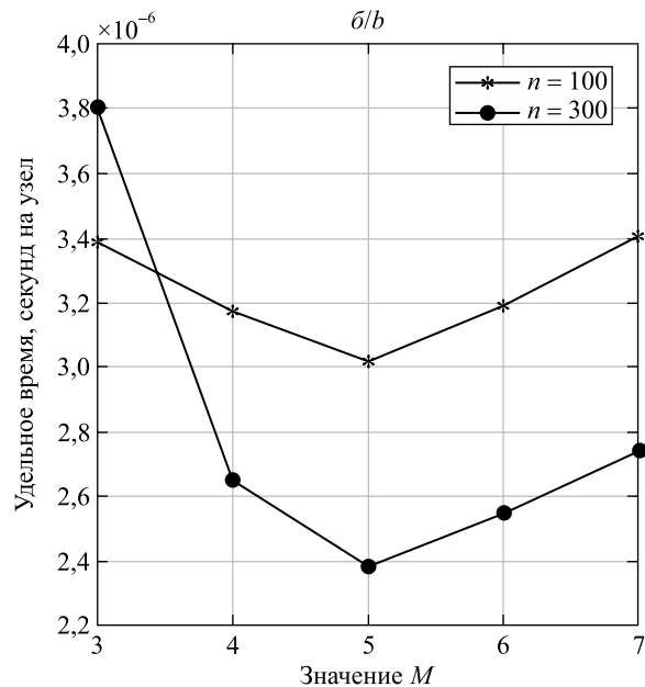
Рис. 2. Зависимость количества внешних итераций метода бисопряженных градиентов (biCG-итераций) (а) и удельных вычислительных затрат алгоритма (б) от количества внутренних итераций ( M ) метода переменных направлений
