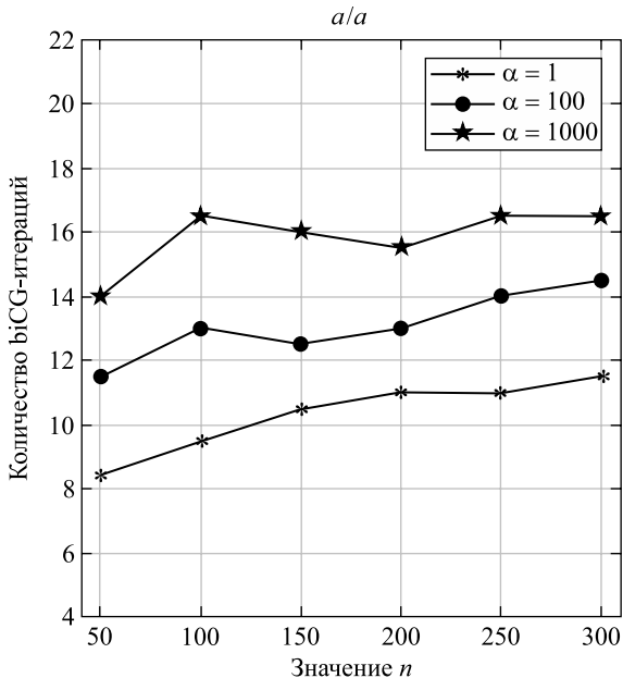
Рис. 3. Зависимость количества biCG-итераций (a) и удельных вычислительных затрат алгоритма (б) от размерности сетки ( n ) при различных диапазонах изменения коэффициента \sigma(x, y)
