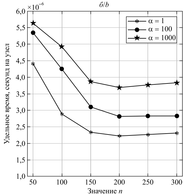
Рис. 3. Зависимость количества biCG-итераций (a) и удельных вычислительных затрат алгоритма (б) от размерности сетки ( n ) при различных диапазонах изменения коэффициента \sigma(x, y)
