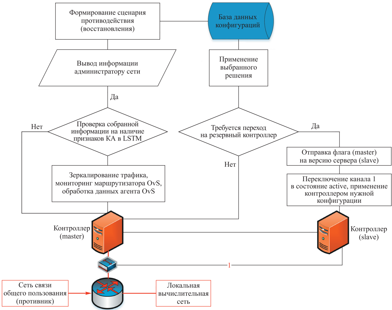
Рис. 8. Блок-схема функционирования сервера системы обеспечения устойчивости SDN
