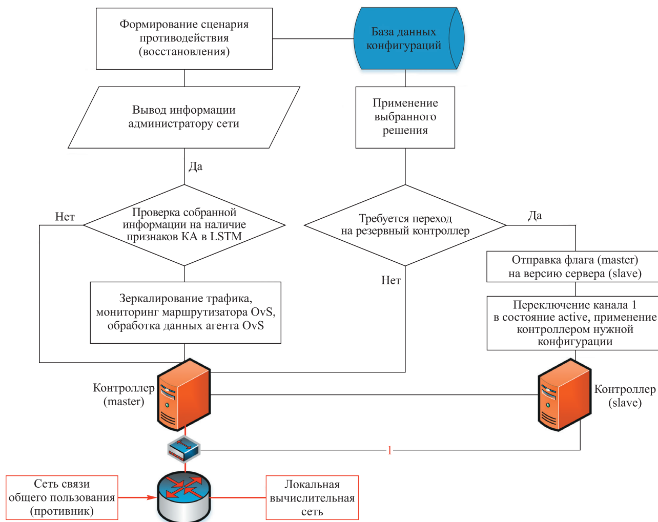
Рис. 8. Блок-схема функционирования сервера системы обеспечения устойчивости SDN
