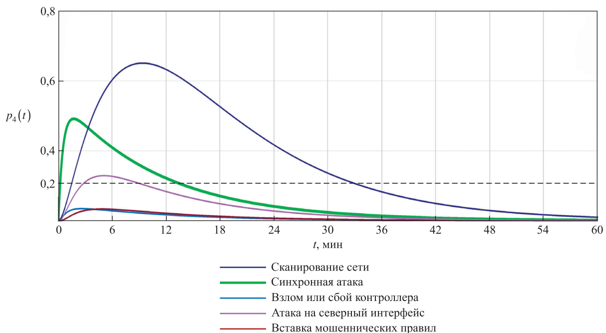
Рис. 4. Зависимость вероятности устойчивой работы SDN от времени реализации КА для структуры 2
