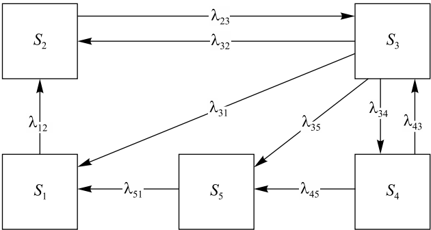
Рис. 1. Граф условных состояний системы передачи данных SDN Fig. 1. SDN state and transition graph
