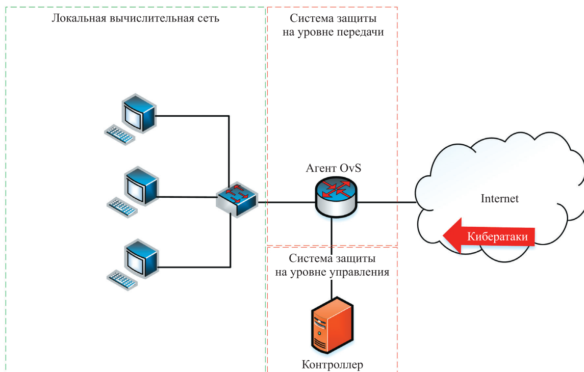
Рис. 6. Вариант предлагаемой структуры построения системы защиты SDN в условиях КА Fig. 6. A variant of the proposed structure of the SDN protection system in cyberattacks conditions
