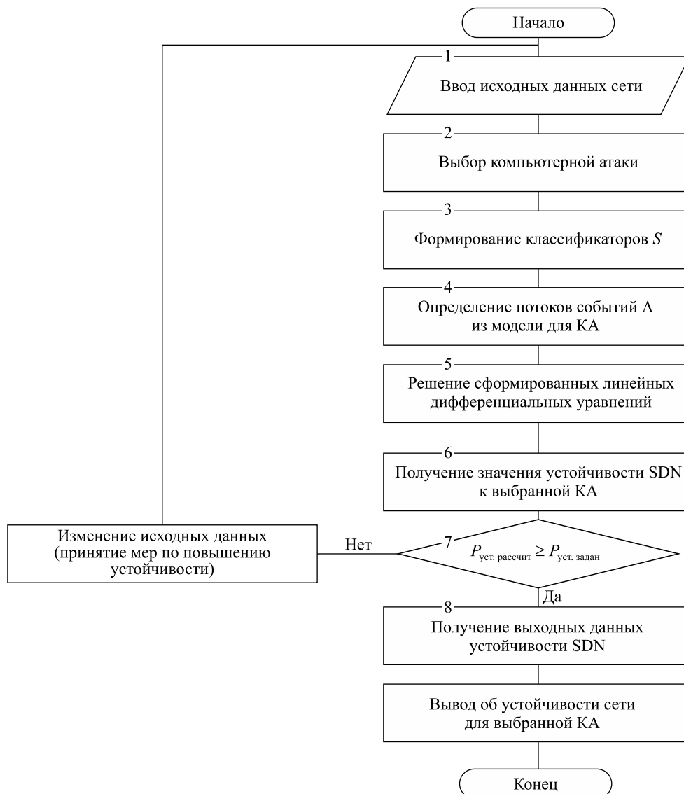
Рис. 2. Блок-схема алгоритма оценки устойчивости SDN в условиях кибератак
