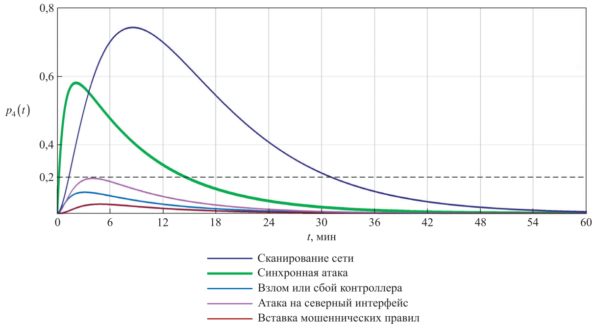
Рис. 3. Зависимость вероятности устойчивой работы SDN от времени реализации КА для структуры 1
