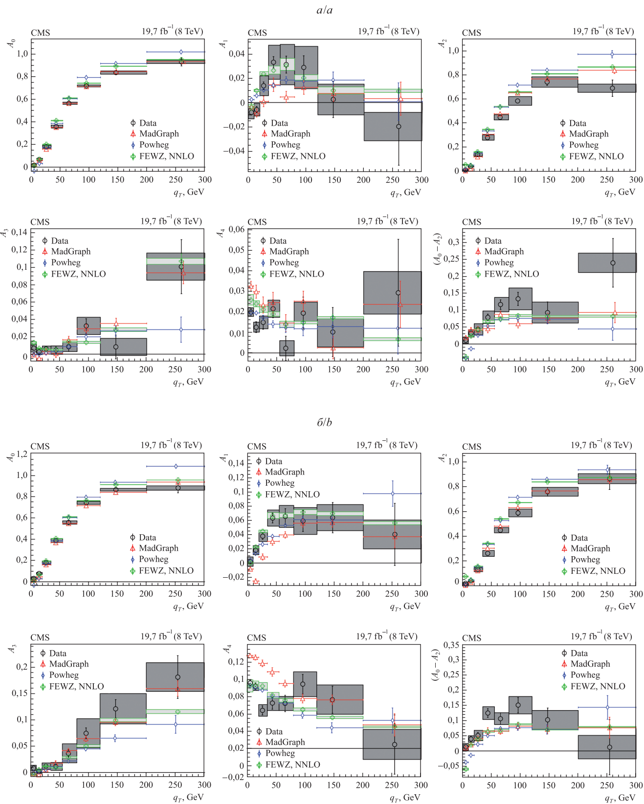
Рис. 5. Сравнение экспериментальных и предсказанных в NLO и NNLO значений угловых коэффициентов A_i и A_0 - A_2 в интервалах быстрот
