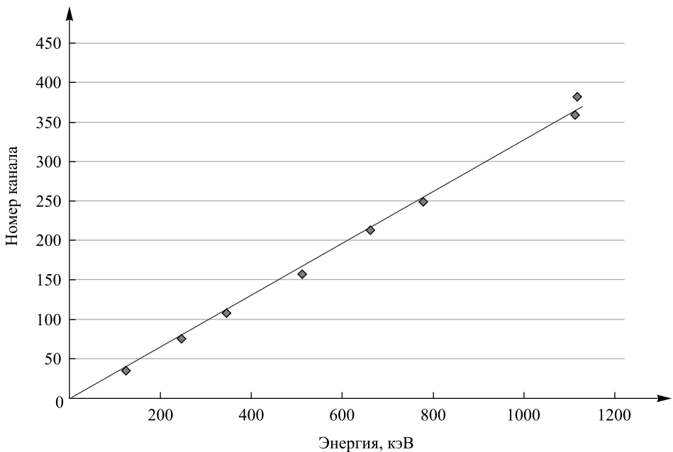
Рис. 3. Градуировочные зависимости номера канала АЦП от энергии гамма-кванта для кристалла \text{Ce}:\text{GAGG} при измерениях с ФЭУ Hamamatsu R3998-100-02 (а) и лавинным фотодиодом (APD) Hamamatsu S8664-1010 (б)
