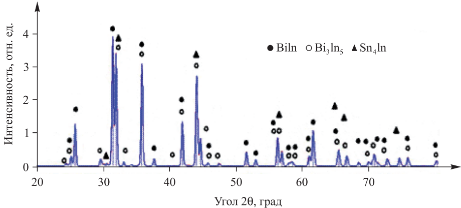
Рис. 1. Дифрактограмма сплава \text{Bi}_{26}\text{In}_{39}\text{Sn}_{35}
