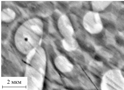
Рис. 2. Микроструктура образца сплава \text{Bi}_{26}\text{In}_{39}\text{Sn}_{35} при различных увеличениях ( а, б )
