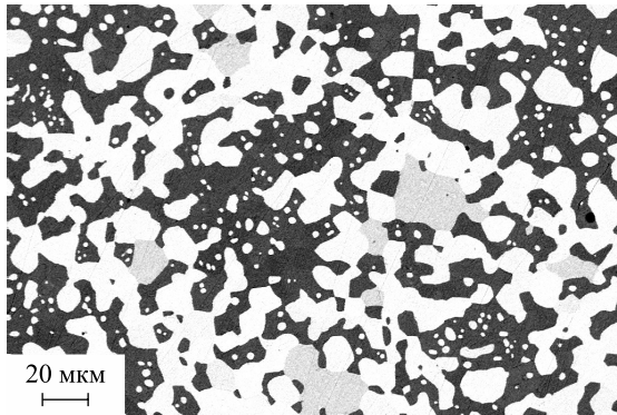
Рис. 2. Микроструктура образца сплава \text{Bi}_{26}\text{In}_{39}\text{Sn}_{35} при различных увеличениях ( а, б )
