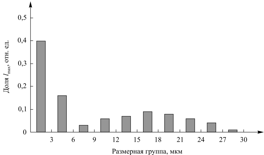
Рис. 3. Распределение максимальных хорд сечений светлых выделений \text{Bi}_{26}\text{In}_{39}\text{Sn}_{35}
