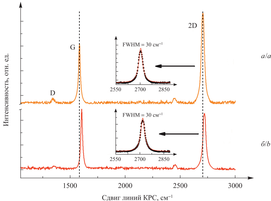
Рис. 1. Характерные спектры КРС экспериментальных образцов графена, выращенного на медной подложке (б) и перенесенного на медную подложку (а).
