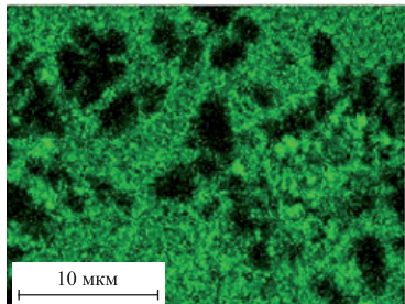
Рис. 4. Распределение Al ( a ) и Si ( б ) по поверхности участка поперечного сечения фольги, полученное в характеристическом рентгеновском излучении
