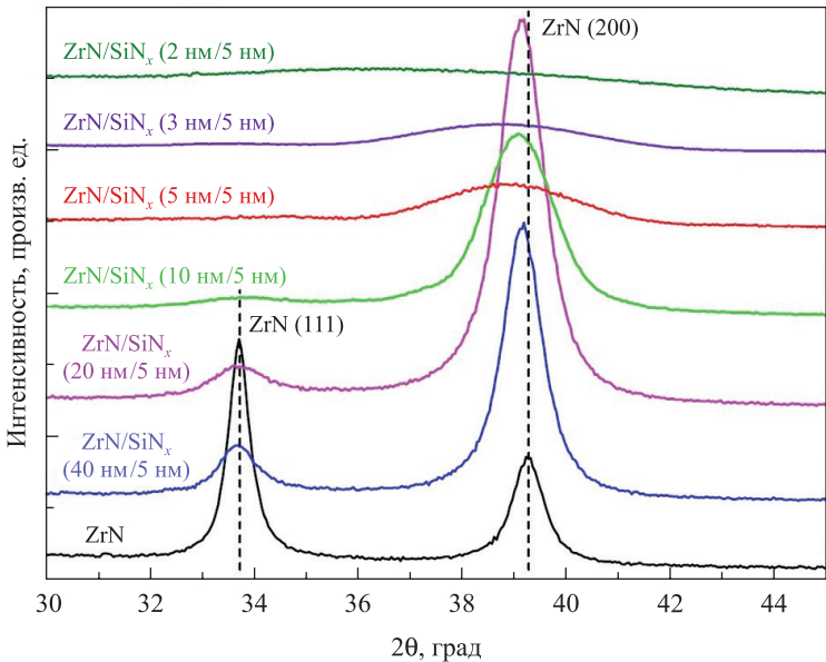
Рис. 3. Дифрактограммы монослойного покрытия ZrN и многослойных покрытий ZrN/SiN x
