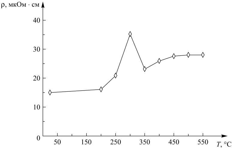
Зависимость удельного сопротивления \rho пленки формируемого силицида Pt от температуры T быстрой термообработки системы Pt – Si Resistivity \rho of the formed Pt silicide film as a function of temperature T during rapid thermal treatment of the Pt – Si system
