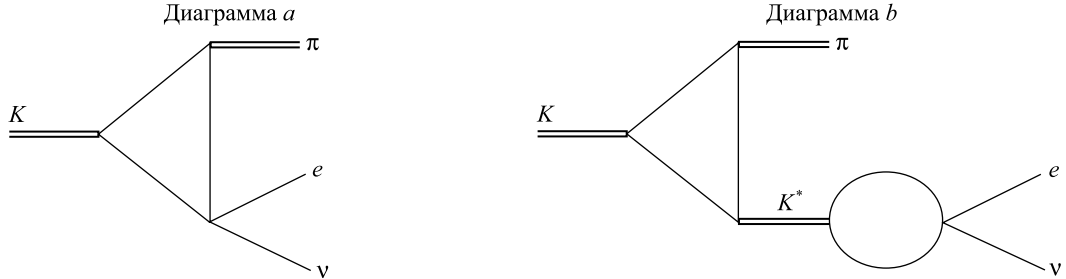
Рис. 1. Диаграммы, описывающие распад K \rightarrow \pi e \nu
