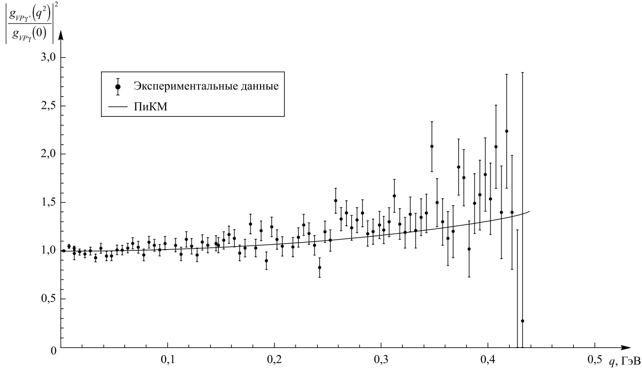
Рис. 2. Поведение формфактора распада \phi \rightarrow \eta \ell^+ \ell^- при различных q
