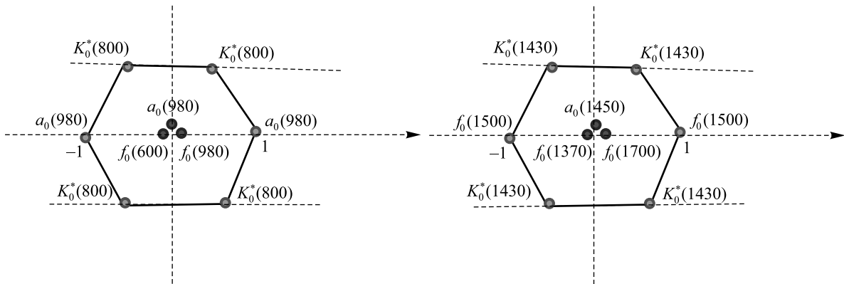
Рис. 1. Нонеты скалярных мезонов.
